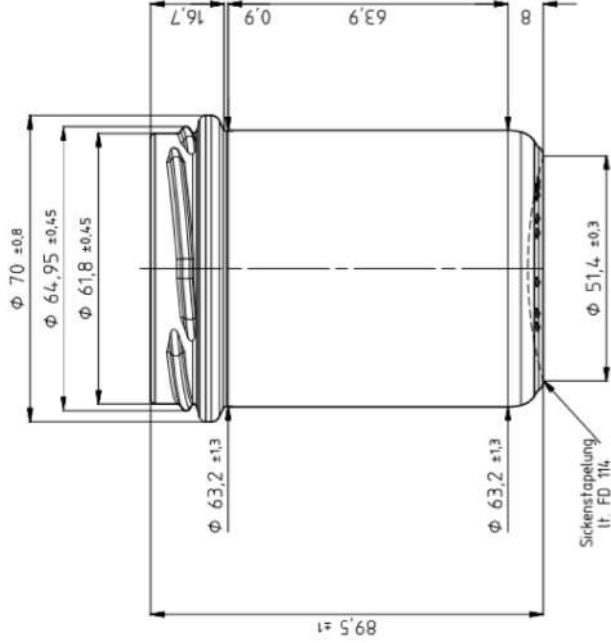
TWIST OFF-Mündung 66 regular nach EN ISO 9100-8
