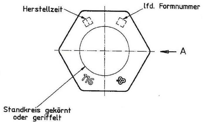
Bodenansicht
